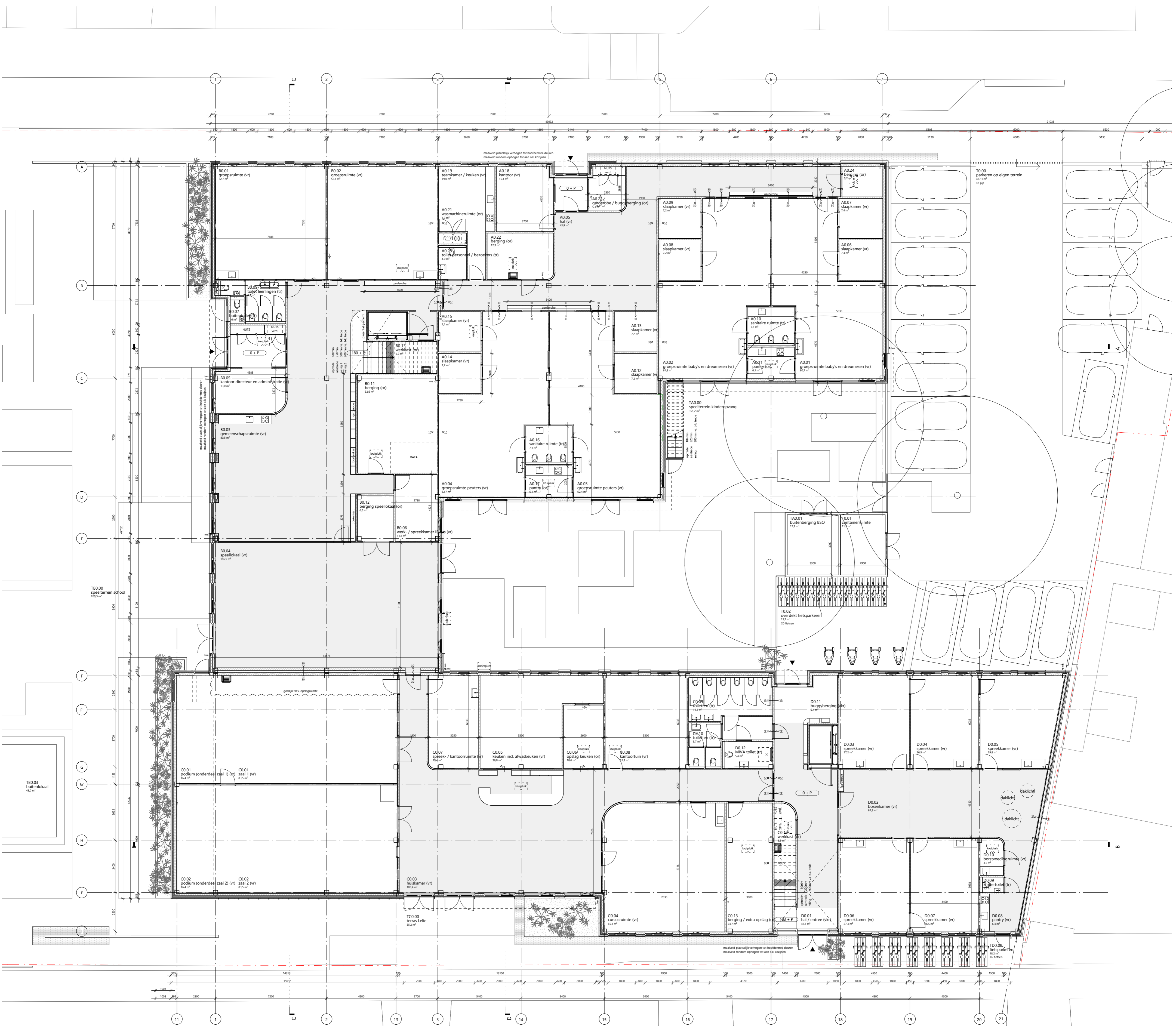
BEGANE GROND
